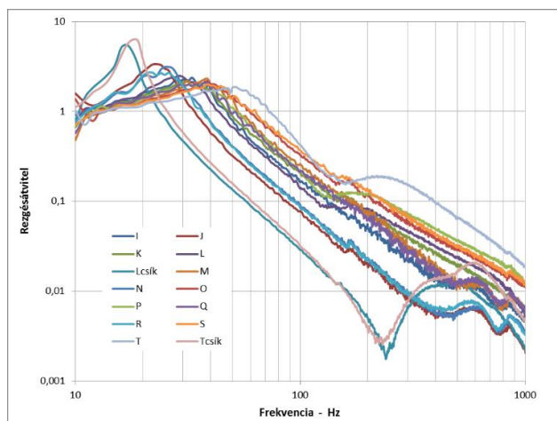
6. ábra. Kevlar kelmékkel megvalósított szendvicsszerkezetek rezgésátviteli függvényének összehasonlítása
